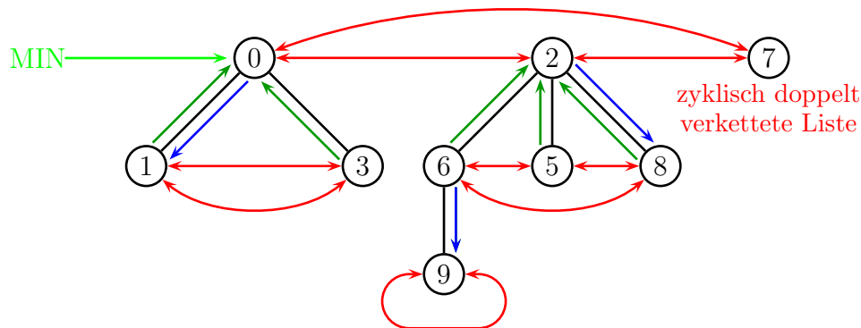
Abbildung 2.58: Beispiel: Fibonacci-Heap
