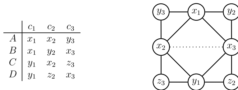
Abbildung 2.20: Beispiel: State-Intersection-Graph
