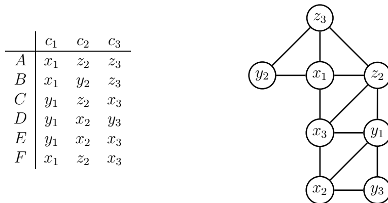
Abbildung 2.16: Beispiel: State-Intersection-Graph
